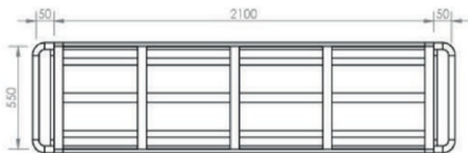
Tampak Atas
